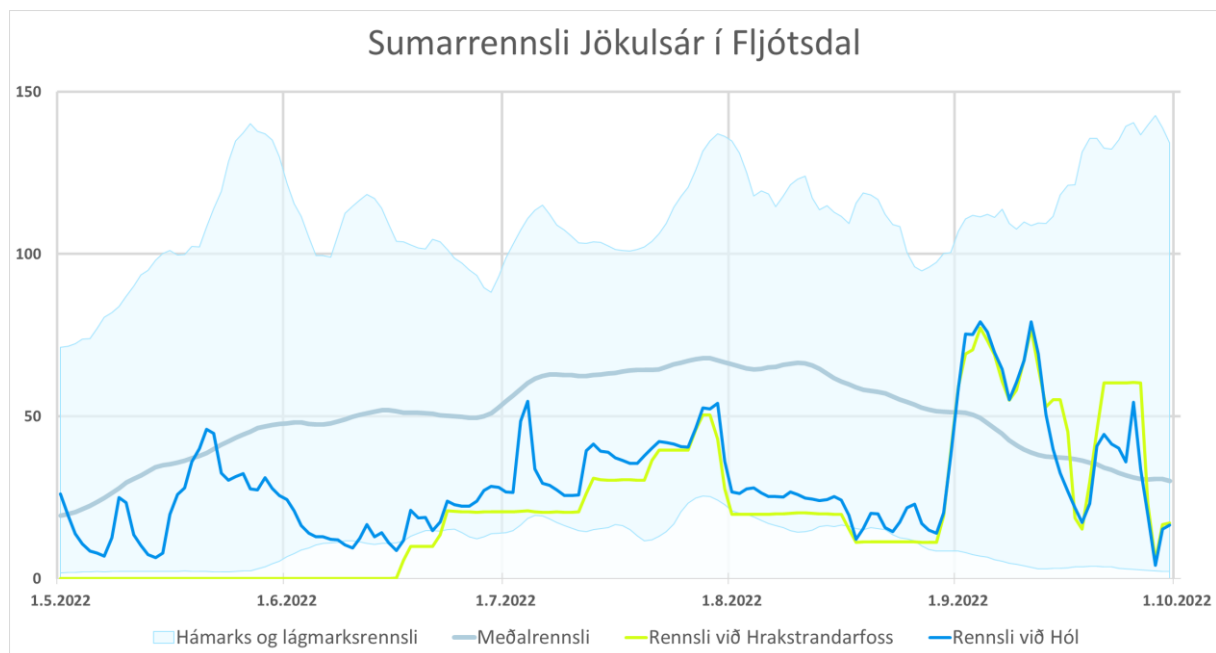
Mynd 2 Sumarrennsli Jökulsár í Fljótsdal 2022
