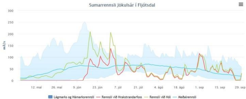
Mynd 10. Sumarrensli Jökulsár í Fljótssdal 2014
