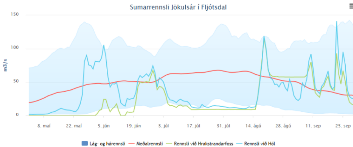
Mynd 8. Sumarrensli Jökulsár í Fljótssdal 2016
