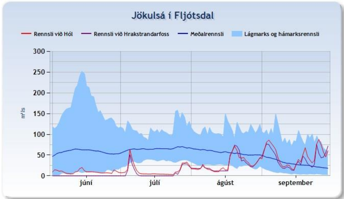
Mynd 13. Sumarrennsli Jökulsár í Fljótsdal 2011
